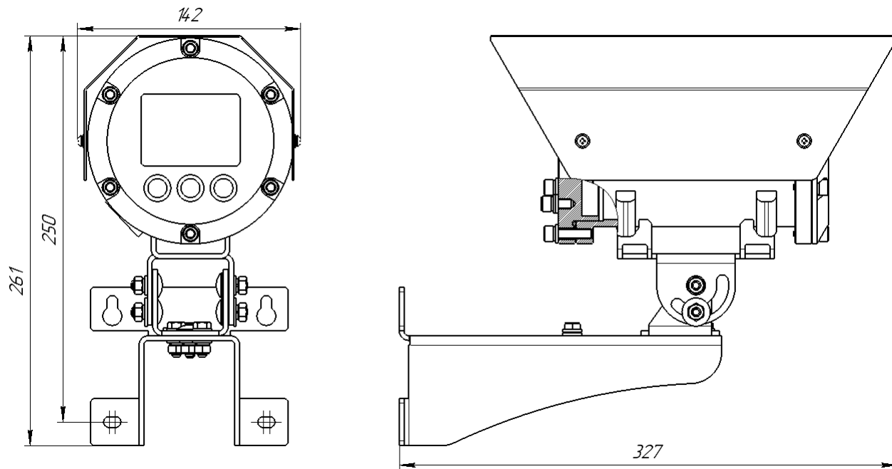
Рисунок А1 – Габаритные размеры видеокамеры АйТек ПРО Н10-Exd
