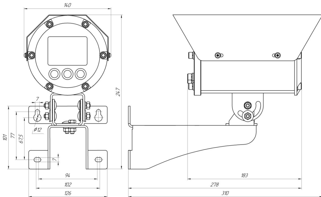
Рисунок А1 – Габаритные размеры видеокамеры АйТек ПРО А-Exd
