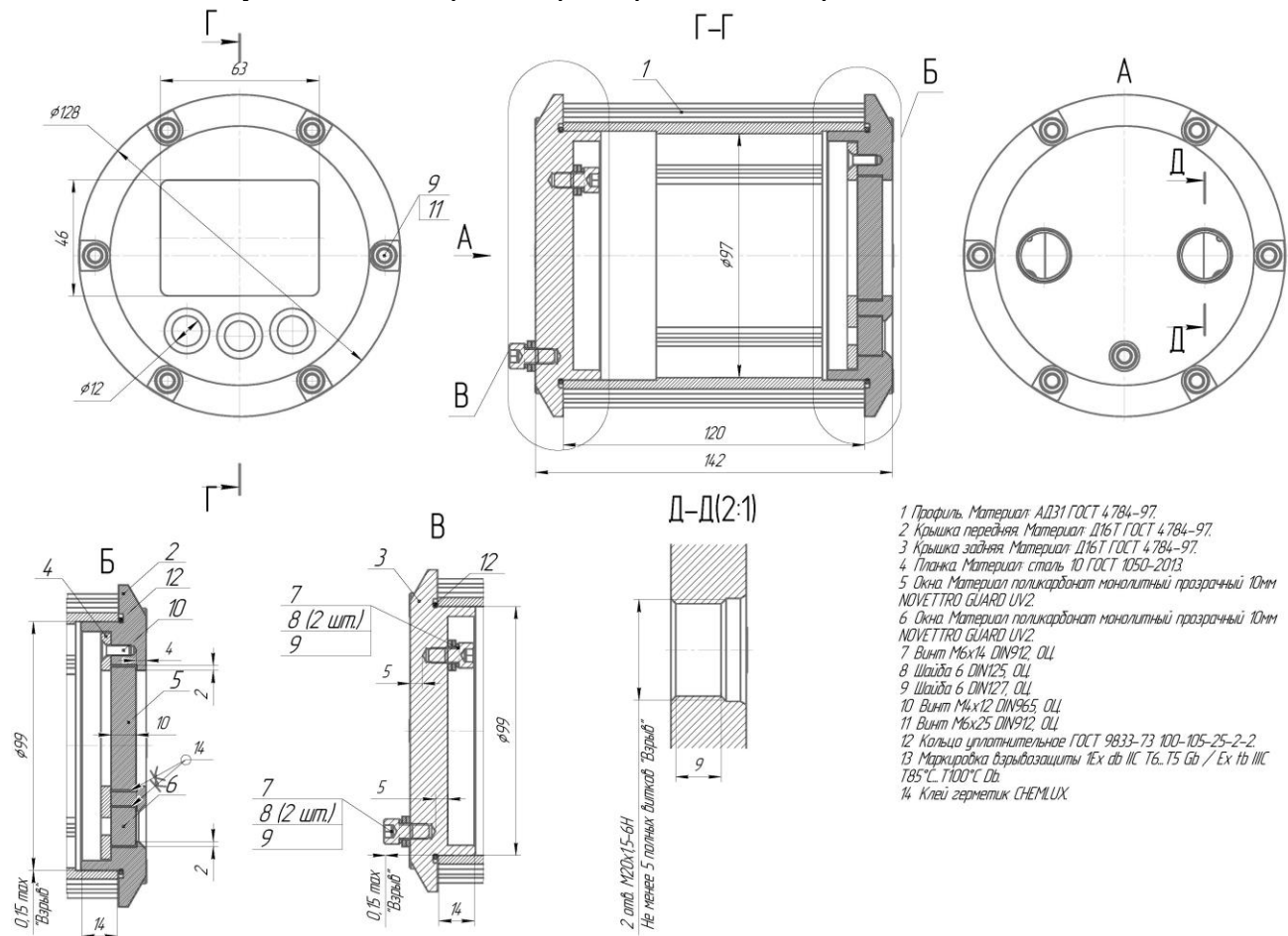
Рисунок А1 – Габаритные размеры видеокамеры АйТек ПРО А-Exd
