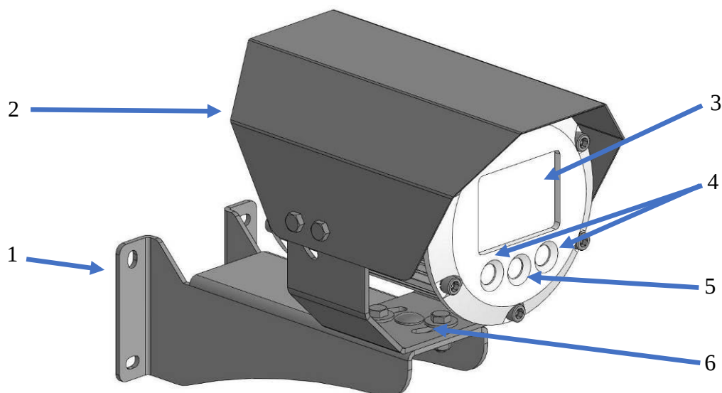
Рисунок 1 – Внешний вид видеокамеры АйТек ПРО A10-Exd
